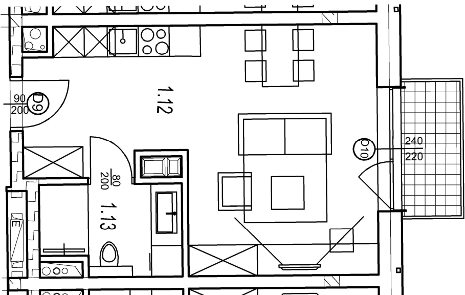
Rzut lokalu 1:75
