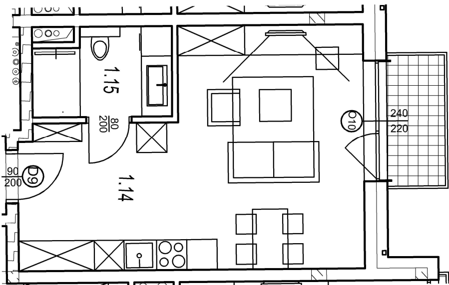
Rzut lokalu 1:75
