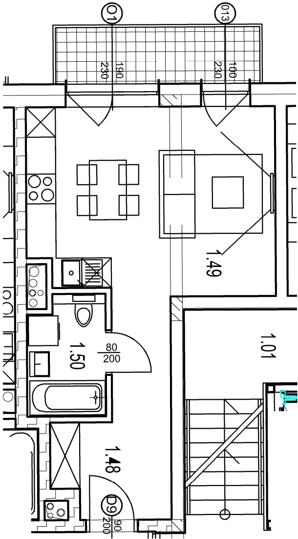
Rzut lokalu 1:75
